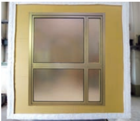
防火試験体:すべり出し段装窓(W1666×H2313)
